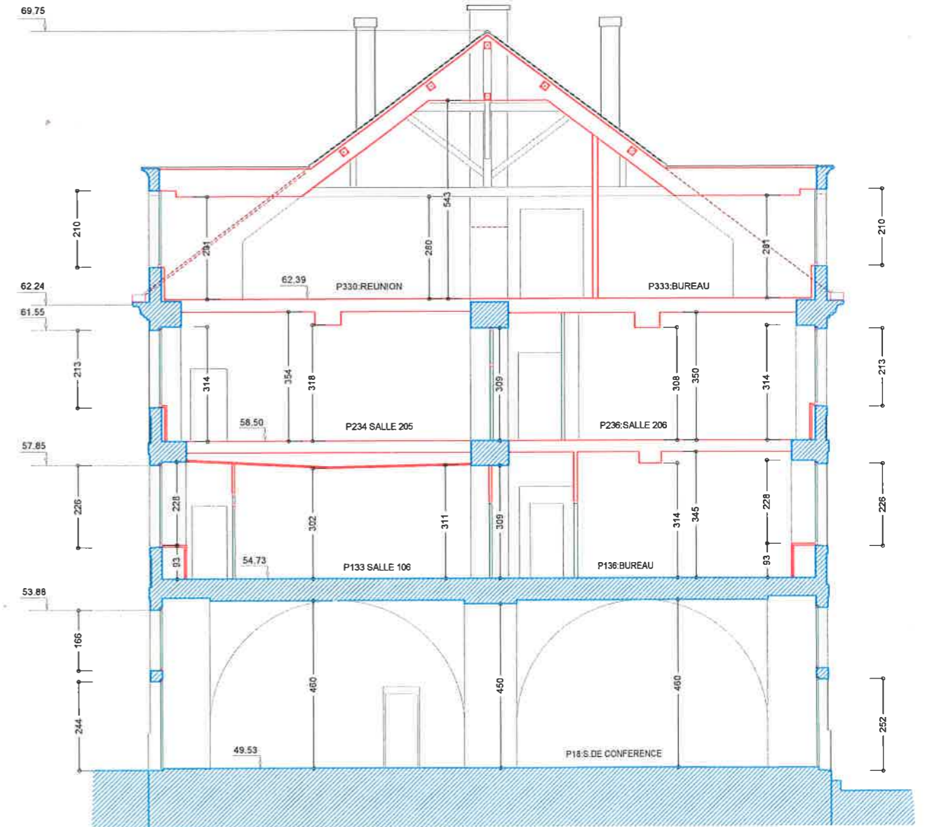
COUPE AA
