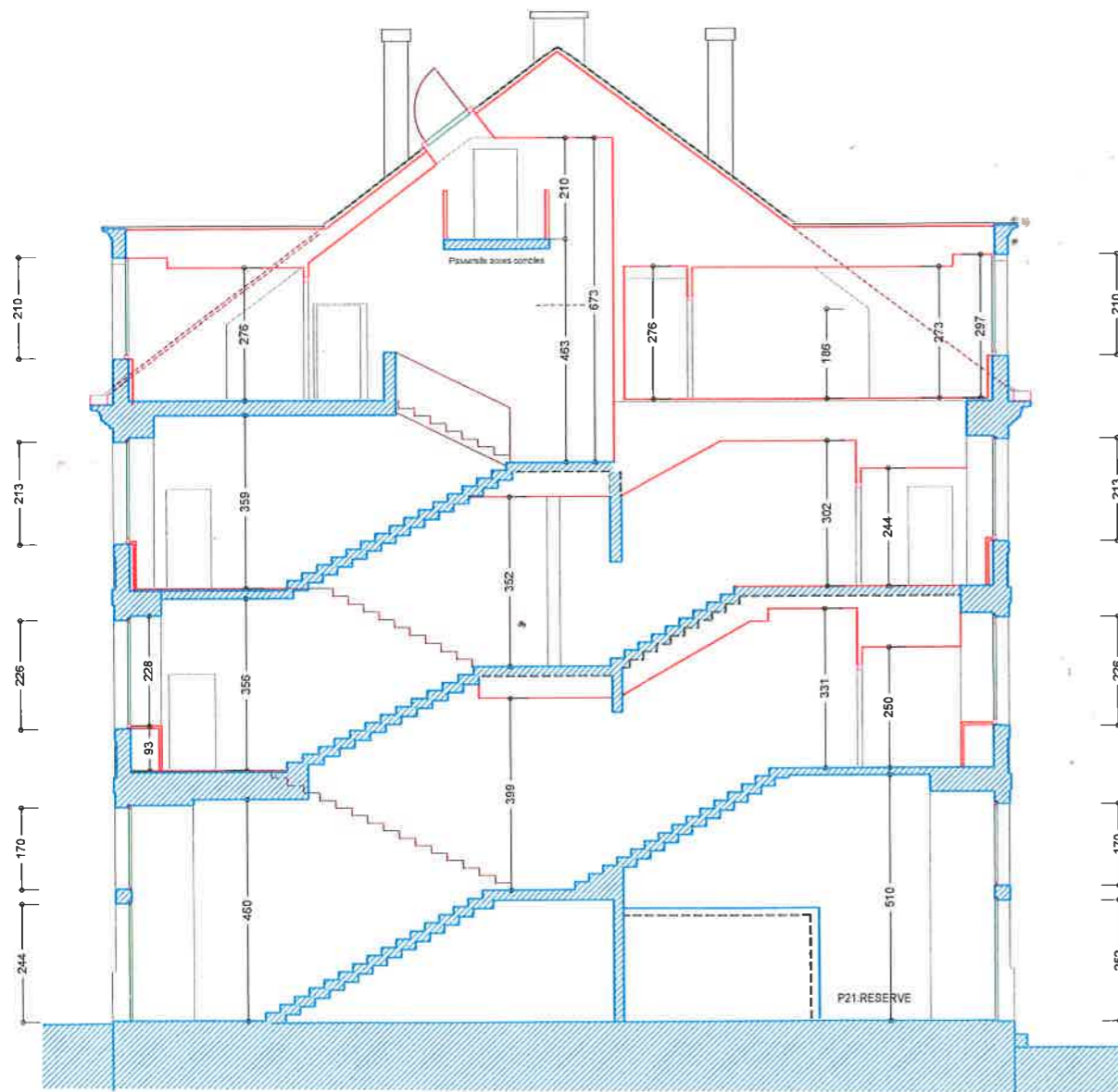
COUPE BB
