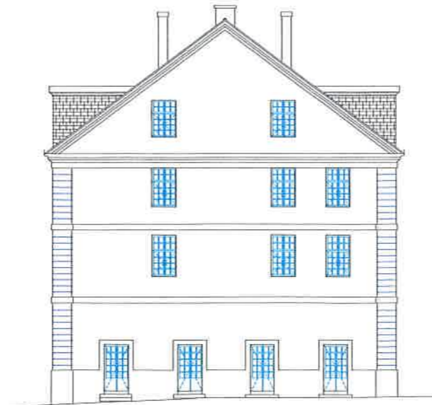
FACADE EST
